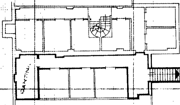
PIANO SCANTINATO h. 2,50
